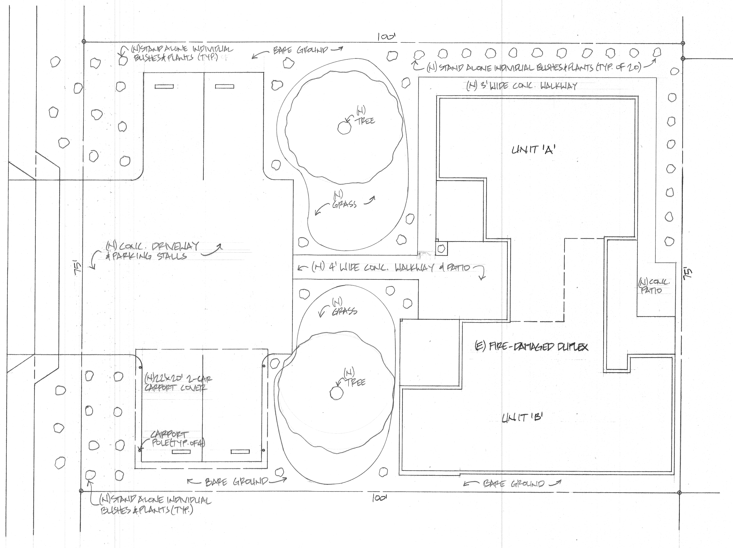
LANDSCAPING PLAN SCALE: 1/8" = 1'-0"
